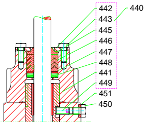
DN 20-150, PN 16-25
