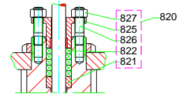
DN 80-150, PN 16-40
